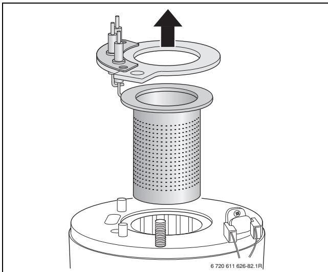
Bild 59 Brenner herausnehmen
