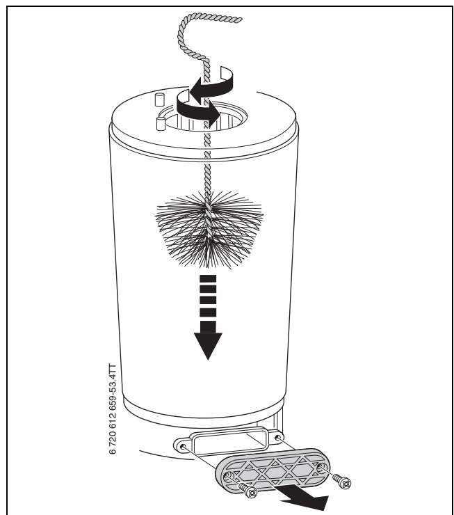
Bild 62 Wärmeblock reinigen
