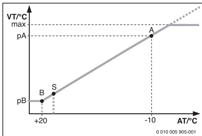
Bild 87 Heizkurve
