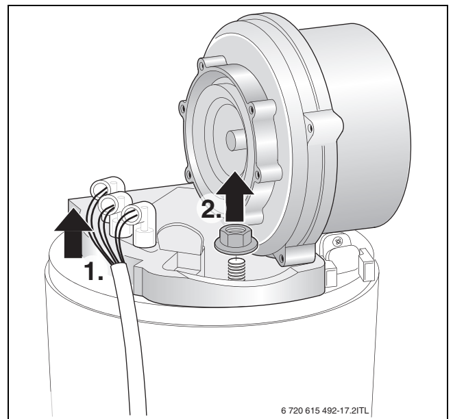
Bild 58 Gebläse herausnehmen
