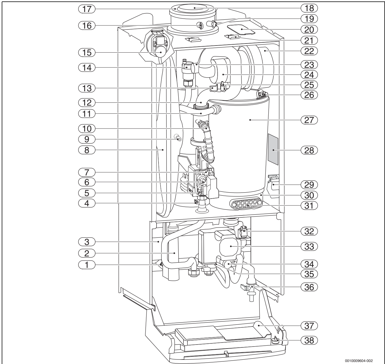
Bild 3 Produktübersicht
