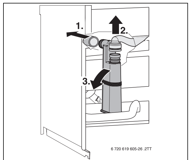
Bild 65 Kondensatsiphon ausbauen
