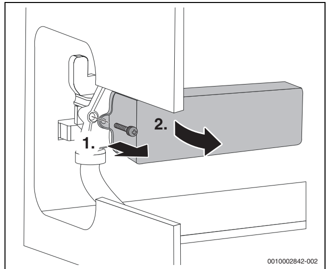
Bild 69 Plattenwärmetauscher ausbauen
