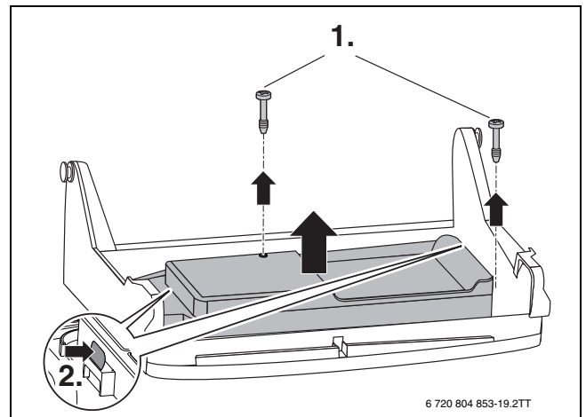
Bild 79 Abdeckung entfernen
