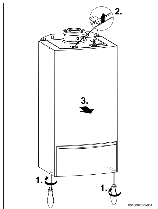
Bild 30 Verkleidung abnehmen
