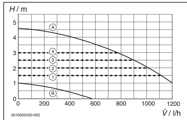
Bild 88 Pumpenkennfelder und Pumpenkennlinien
