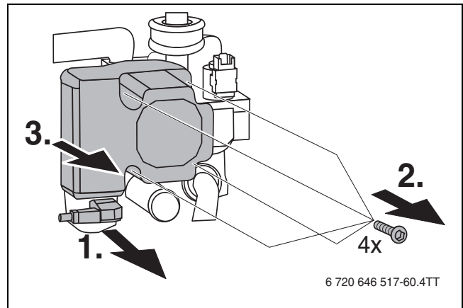
Bild 76 Heizungspumpe ausbauen
