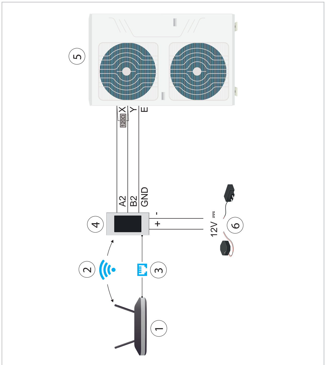
Abb. 25: Anschluss VRF-System
