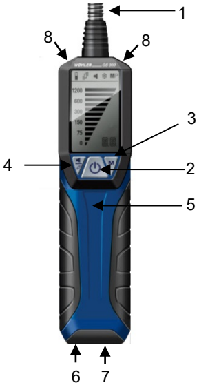
Afb. 23: Gasvoeler
