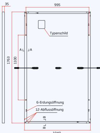
Rückansicht
