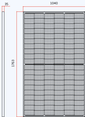
Frontansicht
