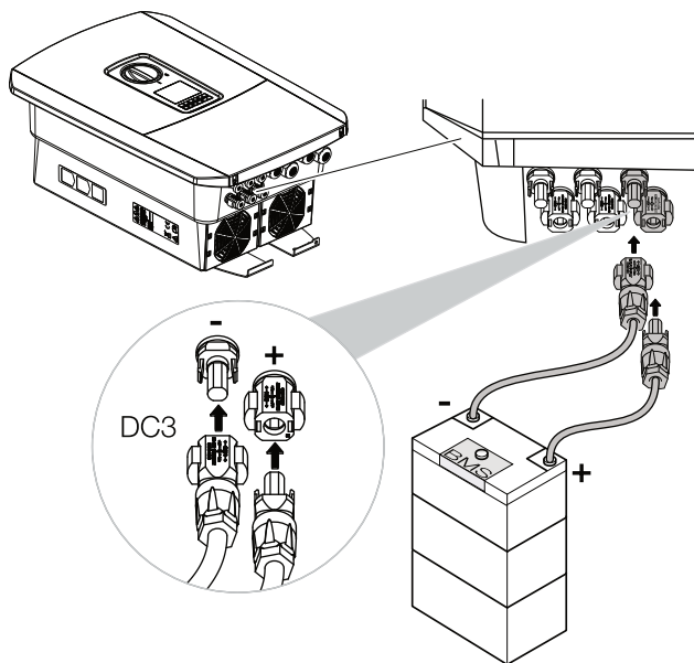
Abb. 38: Übersicht DC-Anschluss Batterie
