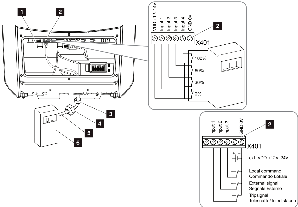
Abb. 31: Anschluss Rundsteuerempfänger !
