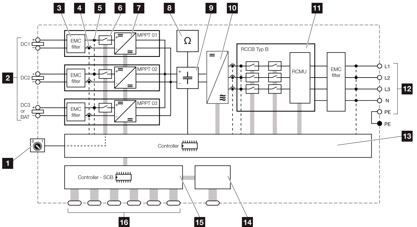
Abb. 75: Blockschaltbild
