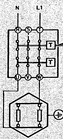
Wechselstrom 230 V ~ Schaltung der Type 2NP 5631.
