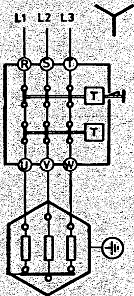
Drehstrom 400 V 3 N ~ Schaltung der Typen 2 NP 5632-2 NP 5636.
