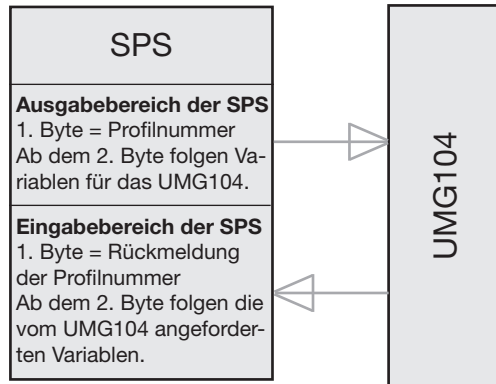
Abb.54.1 Blockschaubild für den Datenaustausch zwischen SPS und UMG104.
