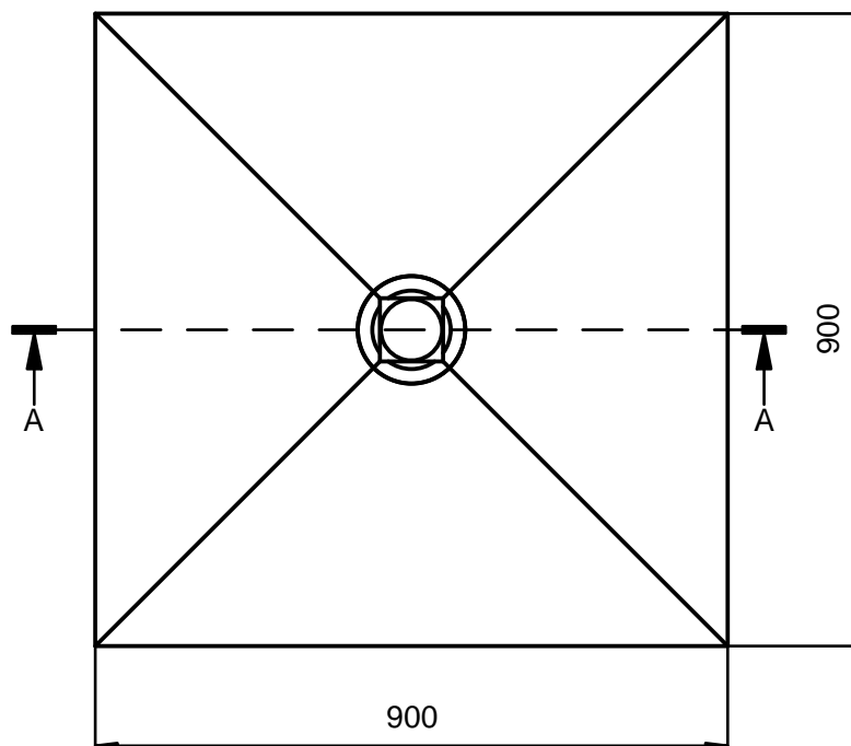
Draufsicht SA32012
