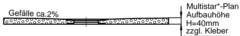
Schnitt A-A
