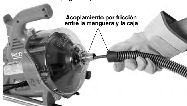
Figura 4 – Alimentación del cable dentro de la manguera-guía
