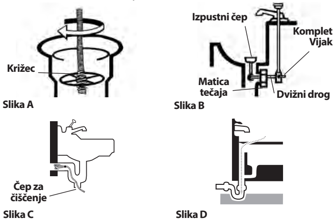
Slika 6 – Dostop do odtoka
