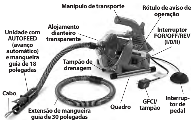
Figura 1 – Máquina de limpeza de tubagens PowerClear
