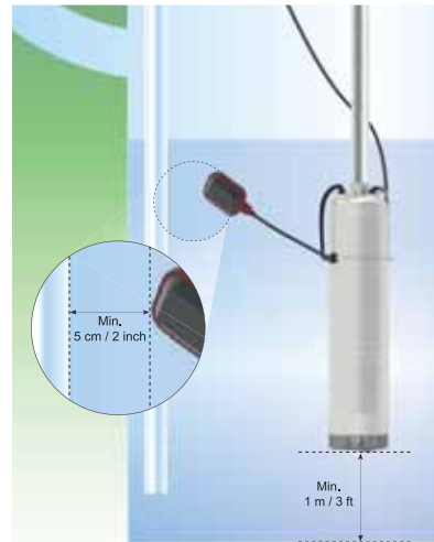
Abb. 3 Mindestabstand zur Wand bei SB-HF-Pumpen; dieses Beispiel zeigt die Installation in einem Brunnen
