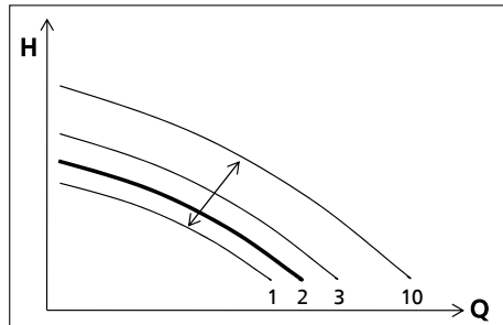
Abb. 25: Funktion Stellerbetrieb, Betrieb auf Drehzahlstufe 2
