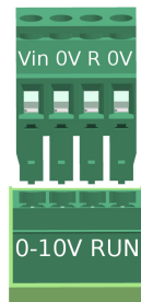
Abb. 11: Klemmenpaar 0-10 V
