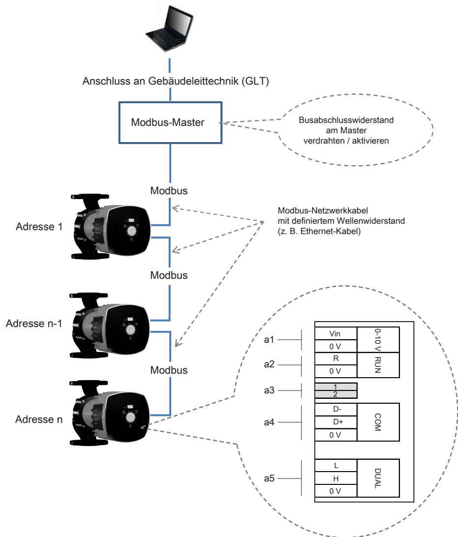
Abb. 13: Modbus-Verkabelung Pumpenaggregate
