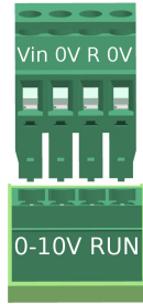
Abb. 12: Klemmenpaar RUN
