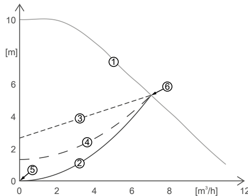
Abb. 23: Eco-Mode und Proportionaldruck am Beispiel Baugröße 25-100
