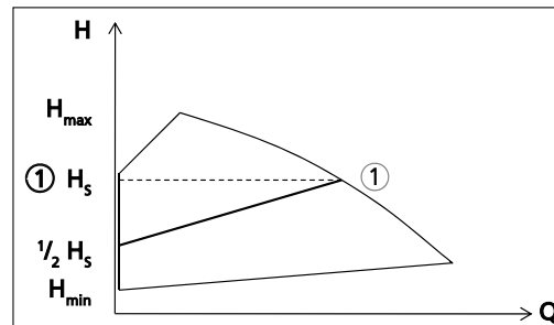
Abb. 21: Funktion Proportionaldruckregelung
