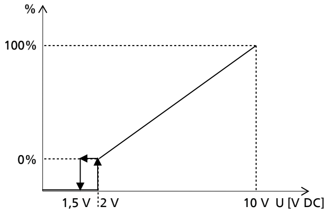
Abb. 27: Analog-Signal 0 - 10V als Sollwertvorgabe an Pumpe
