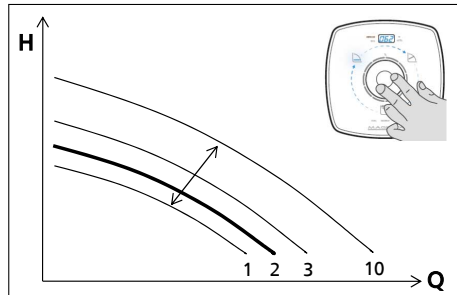
Abb. 26: Einstellung Stellerbetrieb
