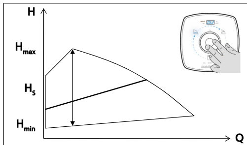
Abb. 22: Einstellung Proportionaldruckregelung
