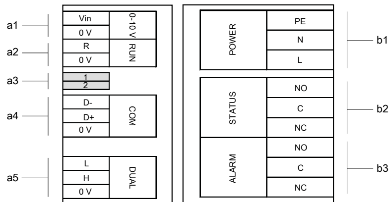
Abb. 30: Elektrischer Anschlussplan
