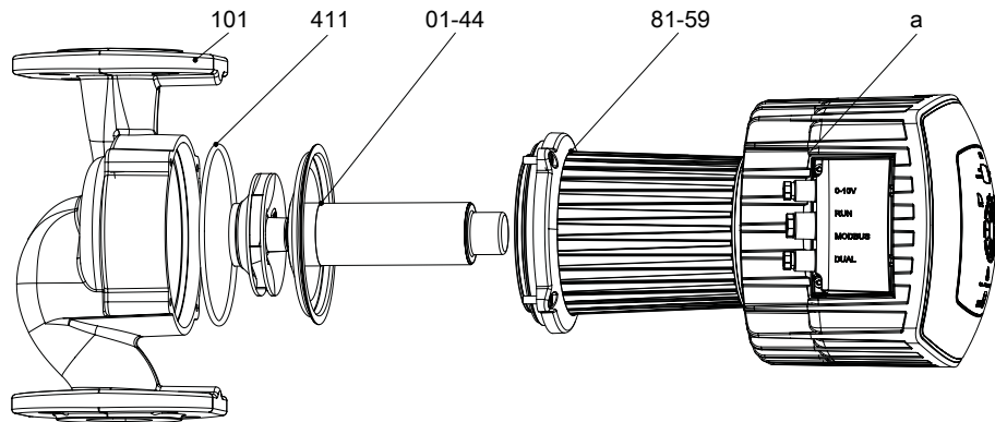
Abb. 29: Explosionsdarstellung
