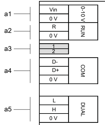
Abb. 16: Klemmenplan Doppelpumpenbetrieb
