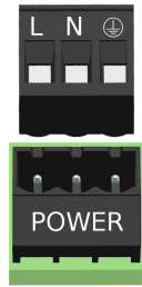
Abb. 8: Netzspannung 1~230 V Wechselstrom +/- 10%, 50 Hz/60 Hz
