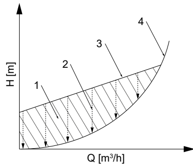
Abb. 28: Prinzip der dynamischen Steuerung
