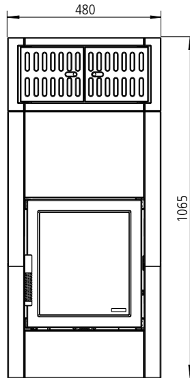
Frontplatte mit Röhrtür und Röhrtüradapter
