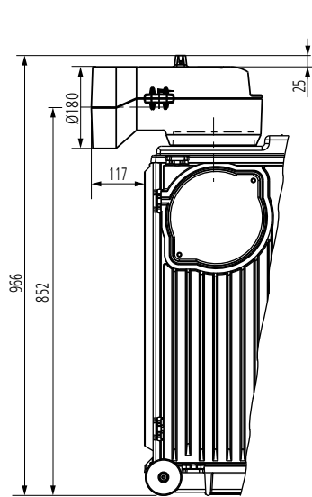
Waagerechter Heizgasstutzen auf BRILLANT
