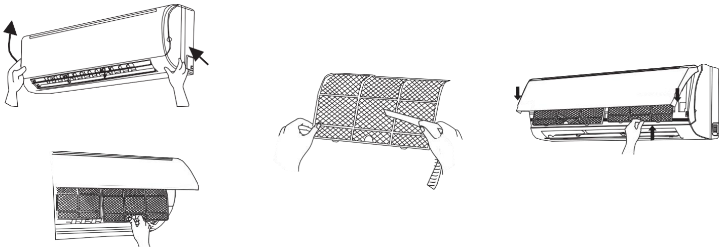
Bild 5: Filterreinigung
