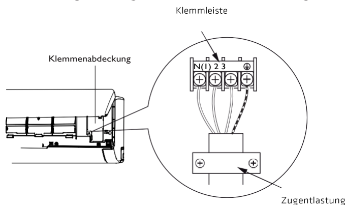
Bild 13: Elektrischer Anschluss Innengerät
