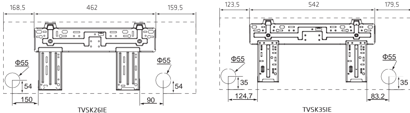
Bild 7: Montageplatte
