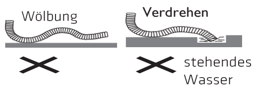
Bild 9: Montage der Kondensatableitung
