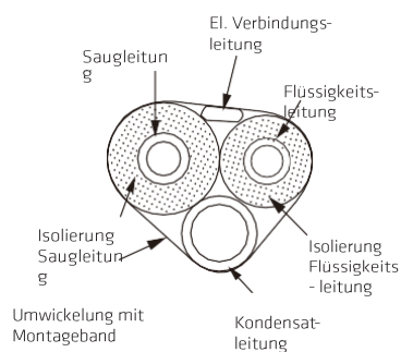
Bild 11: Rohrführung im Querschnitt
