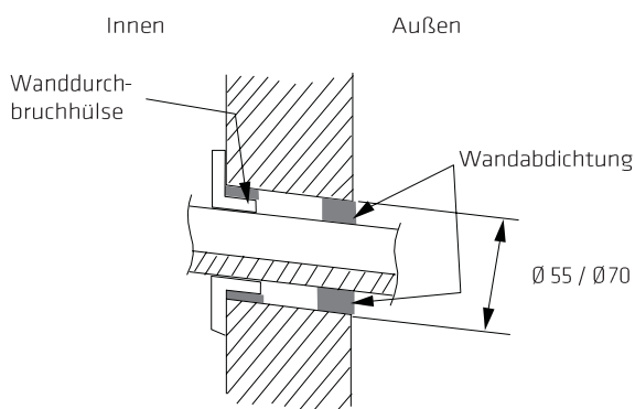
Bild 8: Wanddurchbruch
