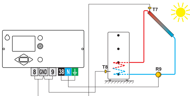
Afbeelding 2- Warmteaccumulator
