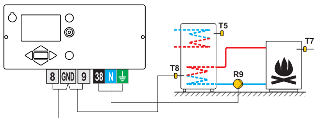
Schéma 1- Chauffe-eau sanitaire
