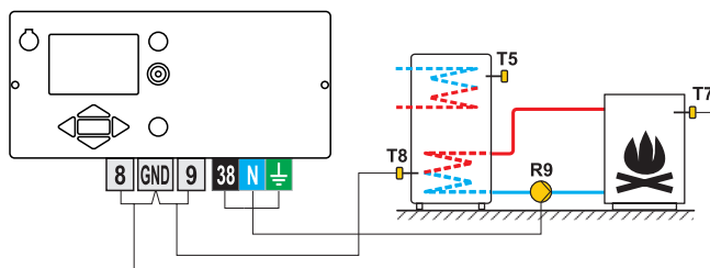
Foto 1 - Dispositivo di riscaldamento dell'acqua sanitaria
