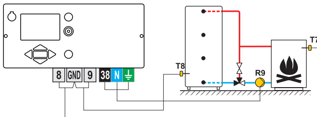
Bild 2- Wärmespeicher
