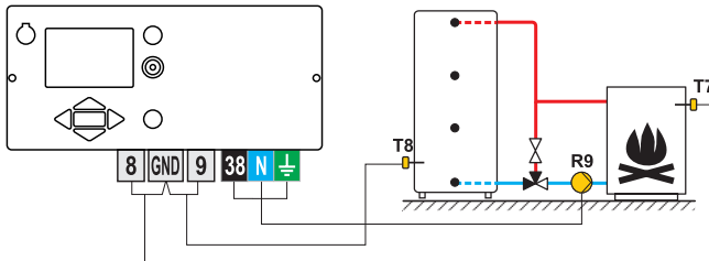
Afbeelding 2- Warmteaccumulator
