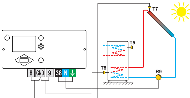
Bild 1- Brauchwassererwärmer
