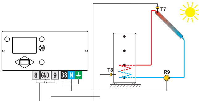
Schéma 2 - Ballon
