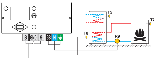
Bild 1- Brauchwassererwärmer
