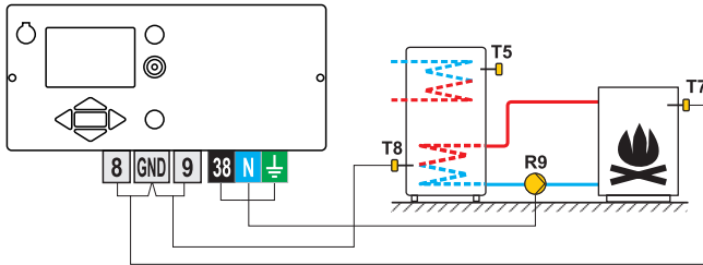
Afbeelding 1 - warmwatertank
