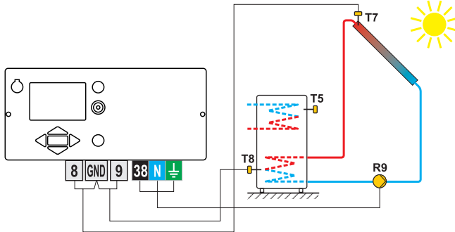
Schéma 1- Chauffe-eau sanitaire
