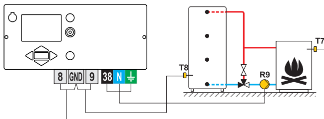
Schéma 2 - Ballon
