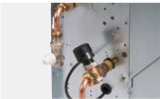
Zweiwege-Ventilbaugruppe, 2-Leiter-System
