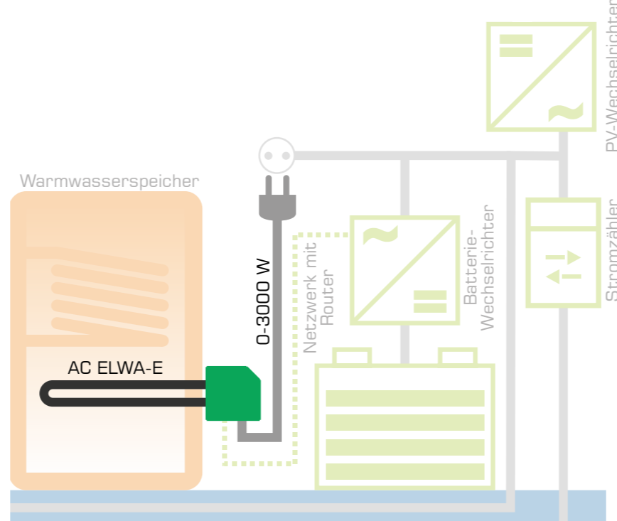
Mit Netzanbindung - mit Batteriespeicher
