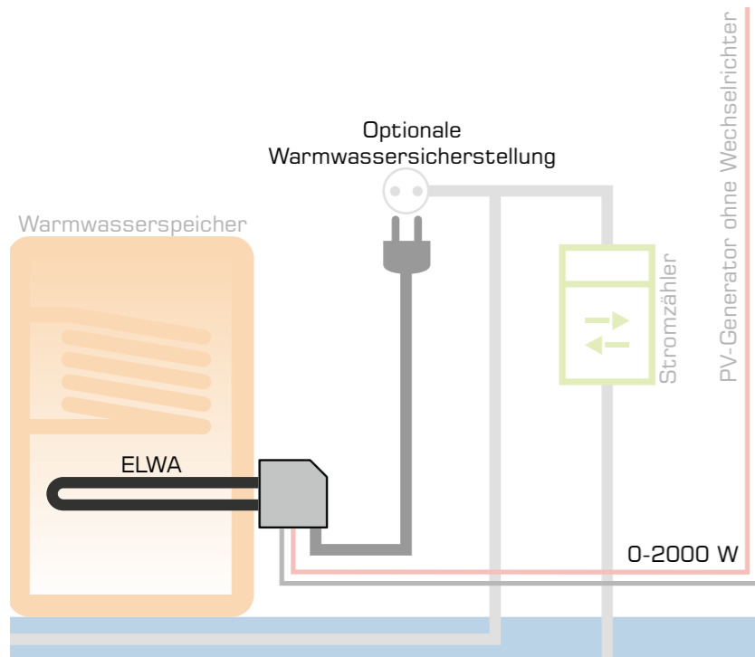
Ohne Netzanbindung - ohne Batteriespeicher
