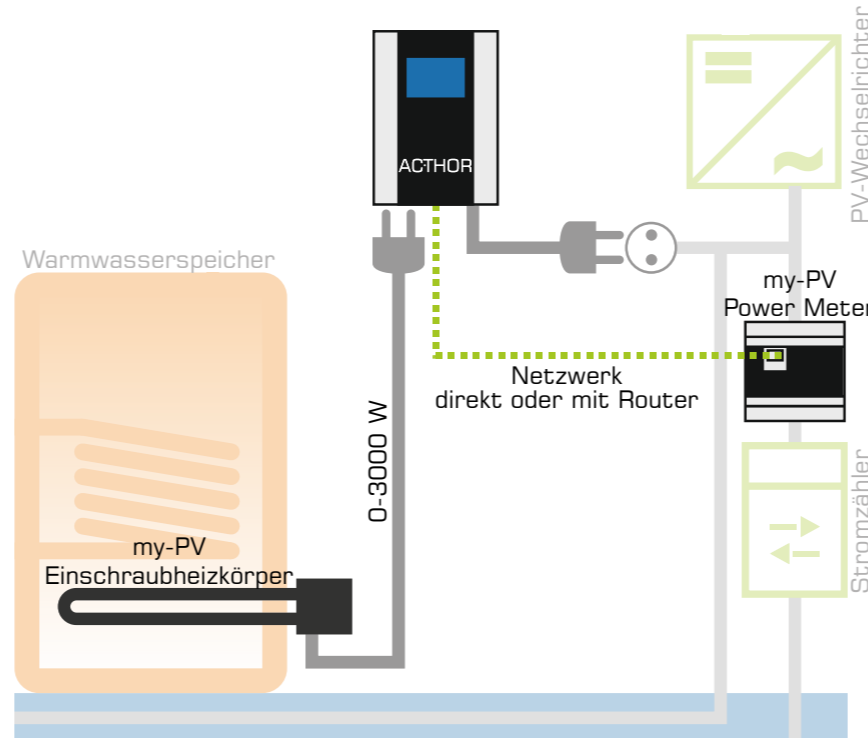
Mit Netzanbindung - ohne Batteriespeicher
