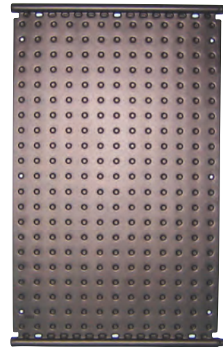
Art.-Nr. 1002 mit integriertem Sammelrohr Ø 40 mm an beiden Schmalseiten Länge 1.360 mm - Breite 820 mm - 1.12 m 2
