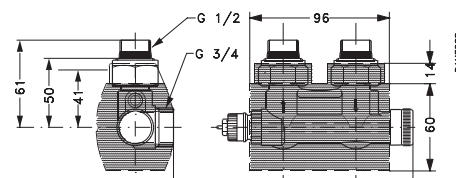
VHS Eckausführung, 1/2 und 3/4" Heizkörperanschluss
