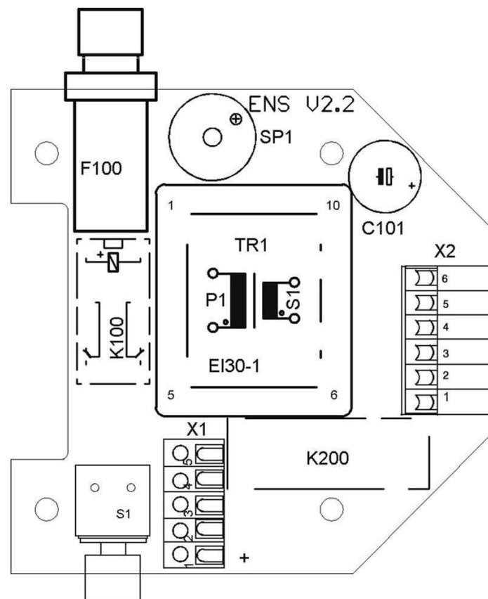
Kontaktbelegung Klemme X1
